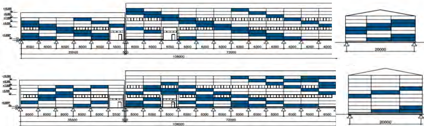
Фасады здания
