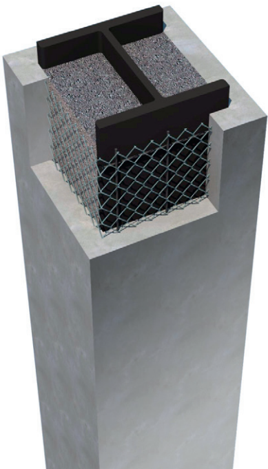
Рисунок 23 Цементно-песчаная штукатурка
