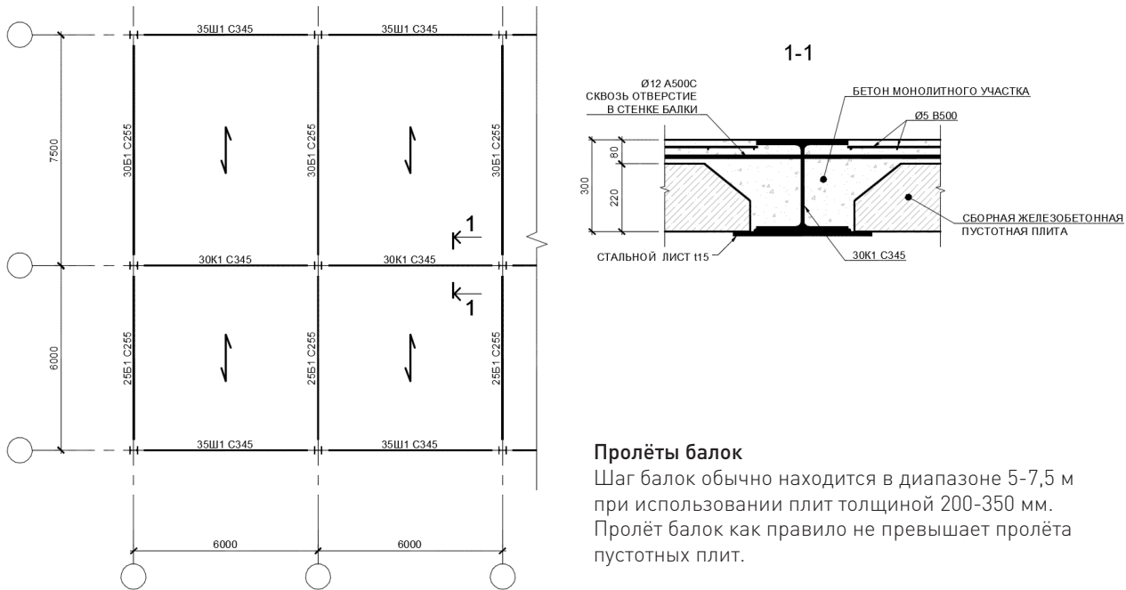
Рисунок 10 Пример расположения балок перекрытия
