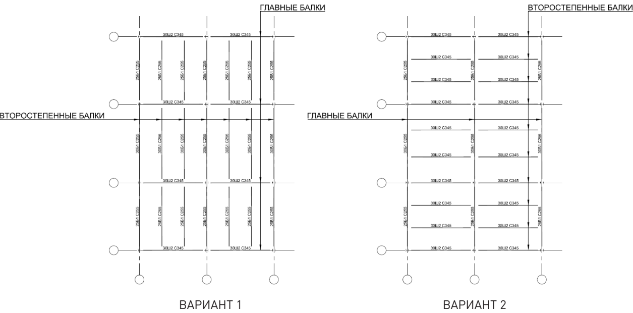
Рисунок 5 Варианты расположения главных и второстепенных балок
