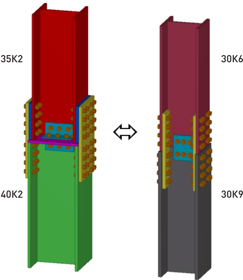
Рисунок 18 Пример оптимизации стыка колонн за счёт назначения единого размерного типа сечений
