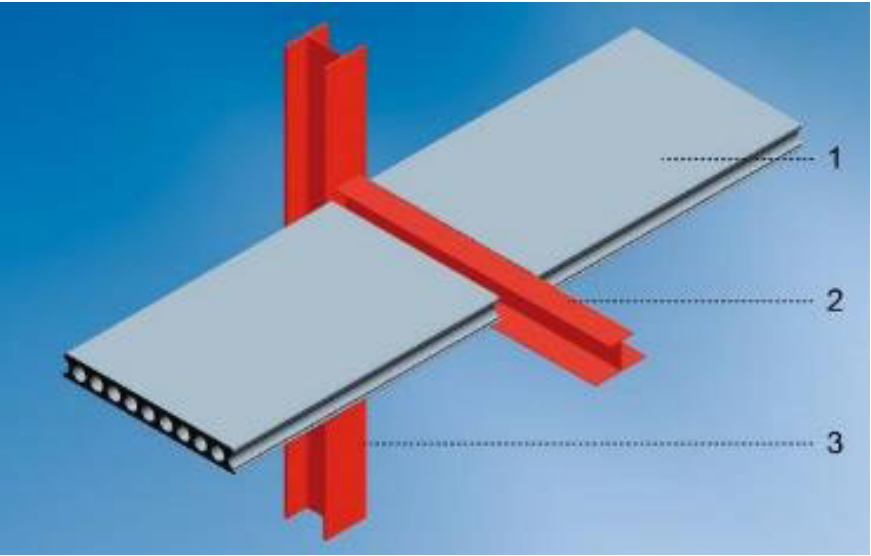
Рисунок 8 Пустотные плиты опираются на нижний пояс стальной балки. 1– сборная железобетонная плита 2 – стальная балка 3 – стальная колонна
