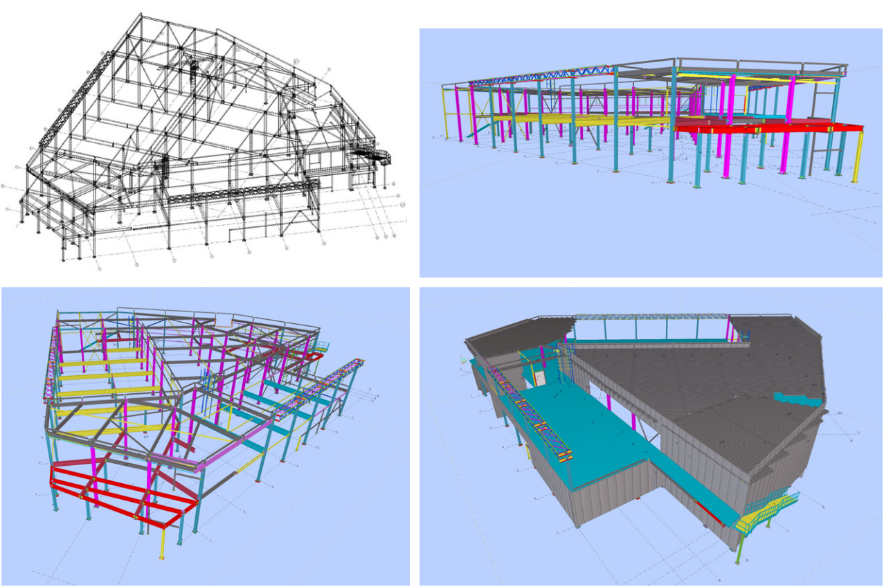
Модели здания, выполненные в Tekla Structures
