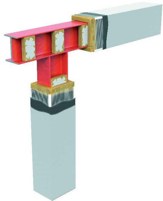
Рисунок 22 Огнезащита минераловатными плитами
