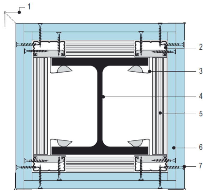
Схема каркасной облицовки стальной колонны с двухслойной обшивкой 1. КНАУФ-профиль углозащитный ПУ 31х31 2. КНАУФ-профиль ПП 60х27 3. Зажим для крепления КНАУФ-профиля ПП 60х27 к колонне 4. Стальная колонна 5. Вставка из КНАУФ-профиля ПП 60х27 на стыках панелей 6. Панель однослойная 12,5 мм 7. Винт самонарезающий (L=45)
